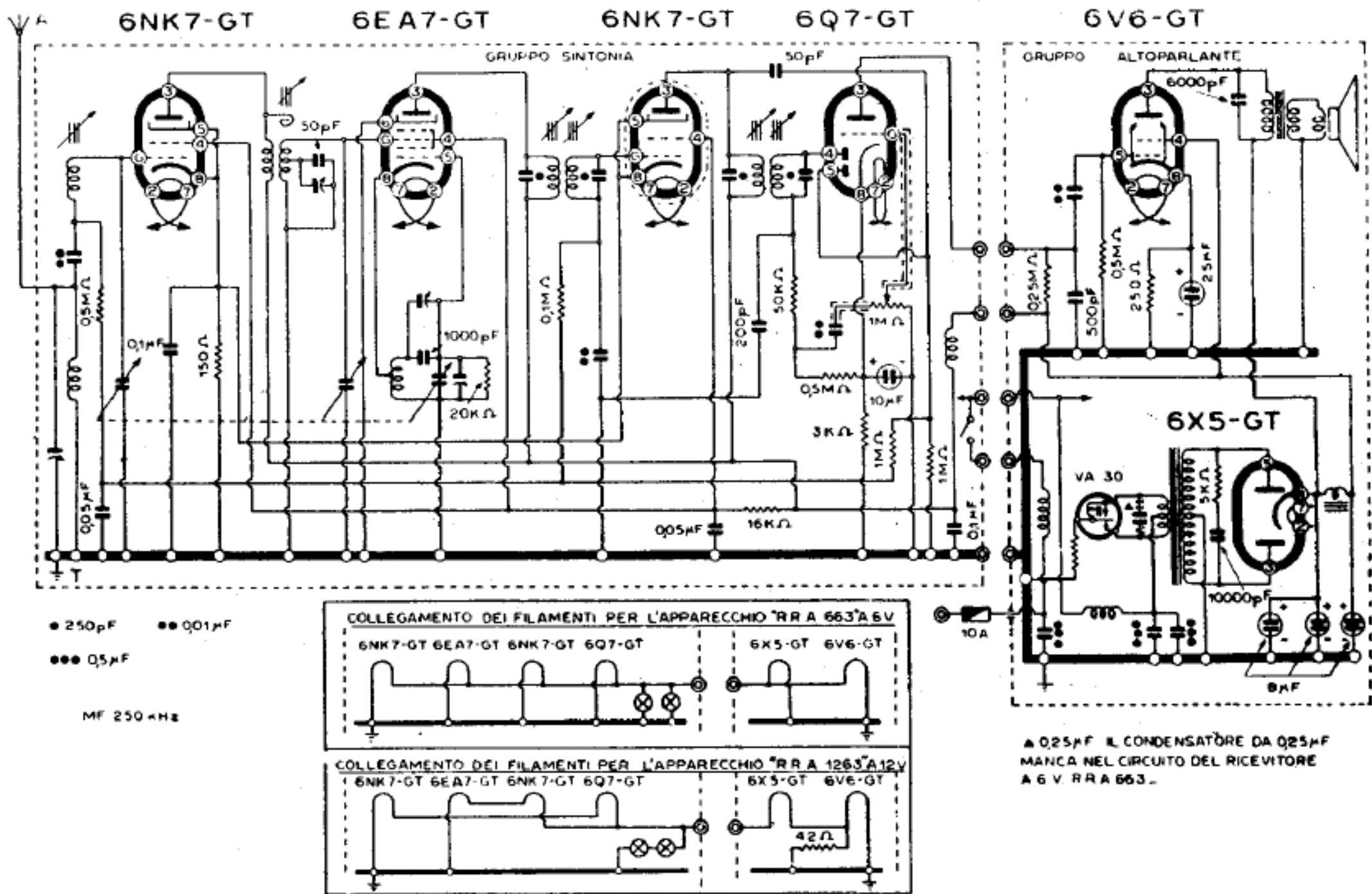
Lo schema elettrico dell'Autovox RRA 663 - RRA 1263.
